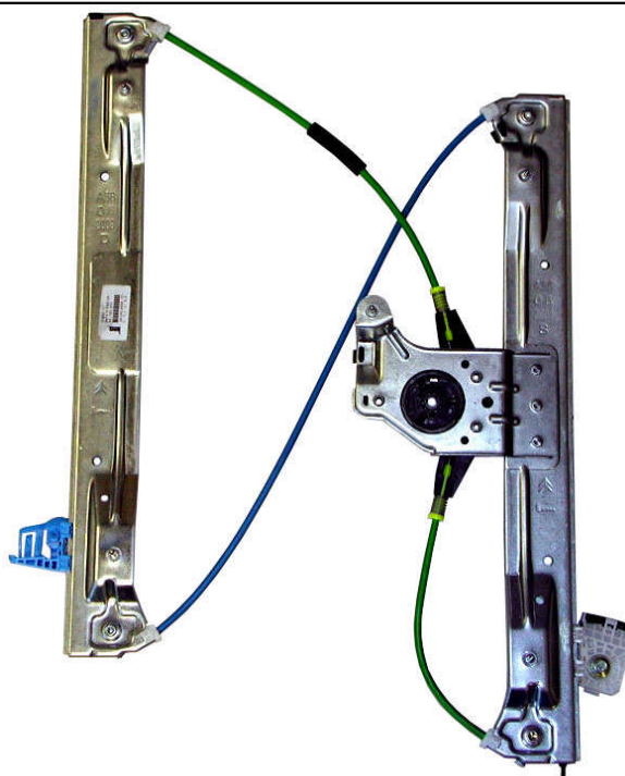
ORIGINAL POWER WINDOW LET ALZACRISTALLI ELETTRICO ORIGINALE SX
